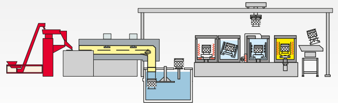
Diskontinuierliches Verfahren
