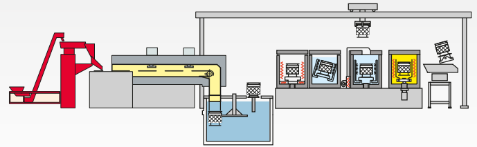
Diskontinuierliches Verfahren
